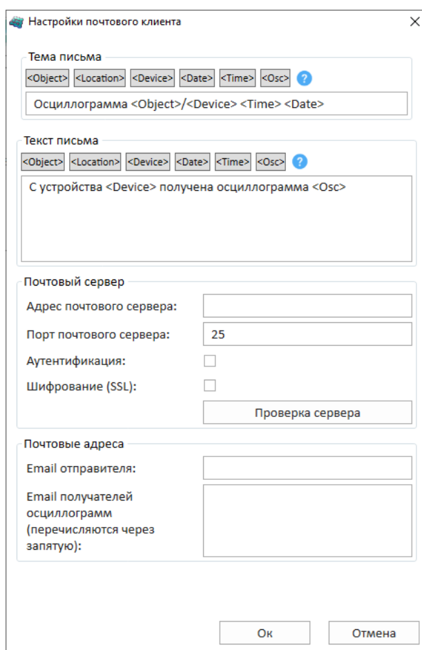
Рисунок 21 – Окно Настройки почтового клиента
