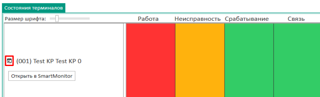
Рисунок 8 – Запуск программы Smart Monitor
