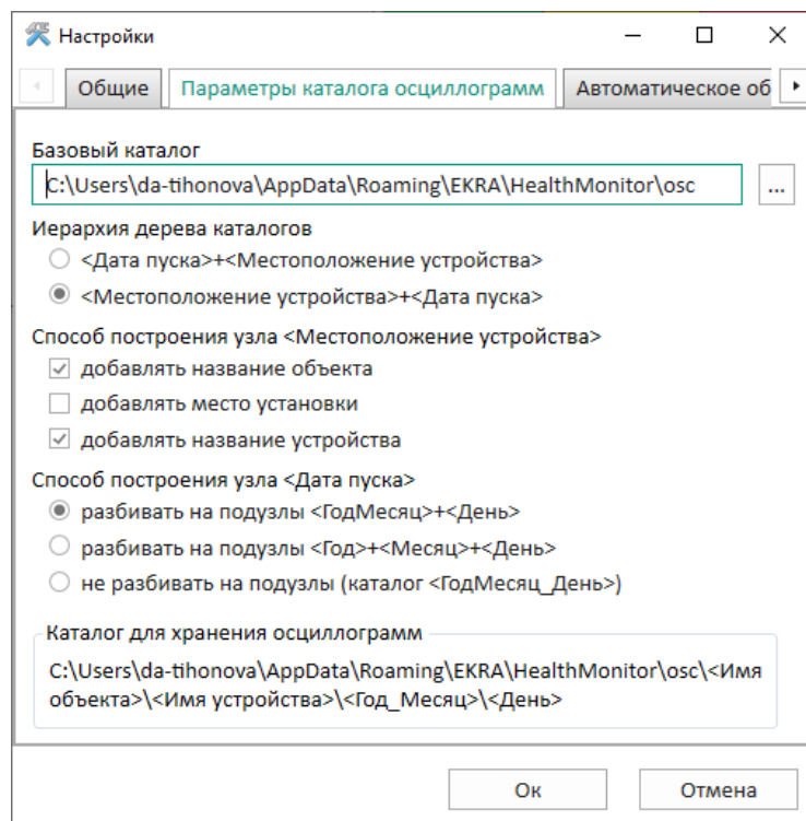
Рисунок 16 – Вкладка Параметры каталога осциллограмм
